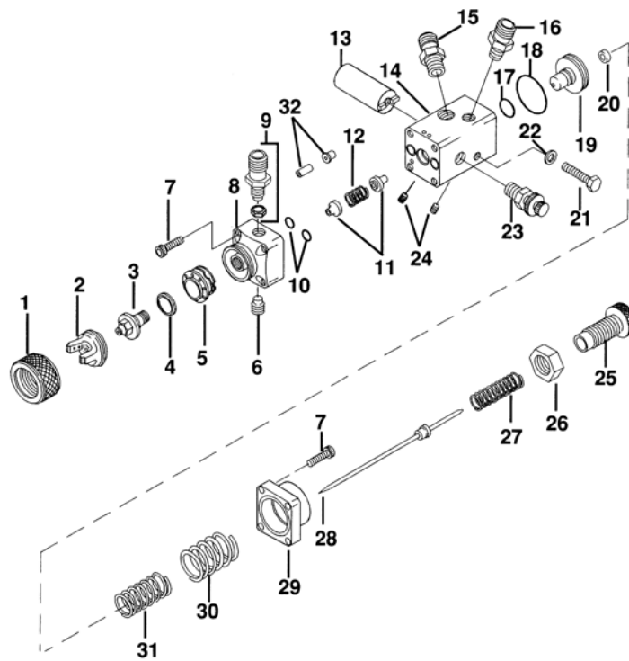
図. 5 ガン分解図
