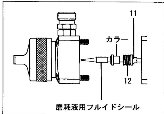
No.32詳細図
